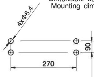
Dimensiuni de montaj/ Mounting dimensions
